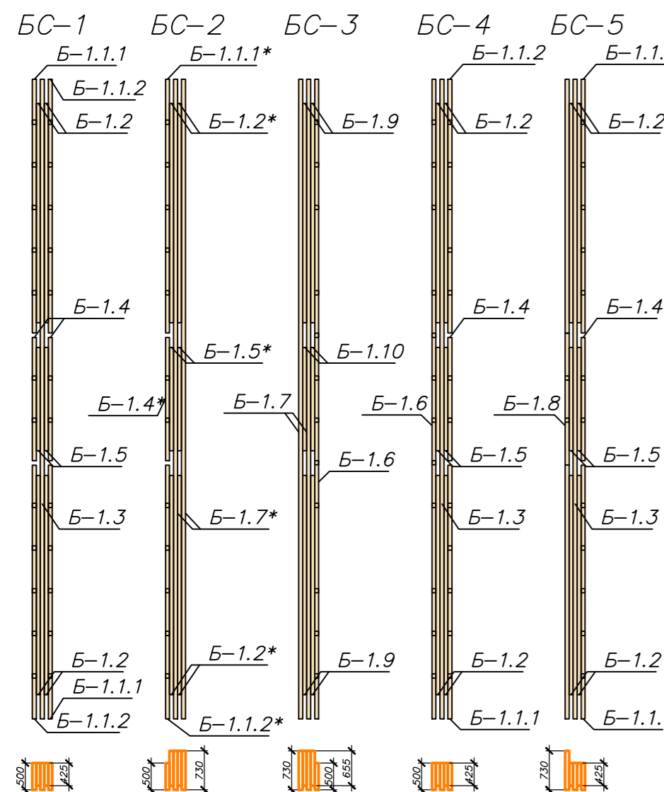
Схема расстановки балок в составных балках перекрытий
